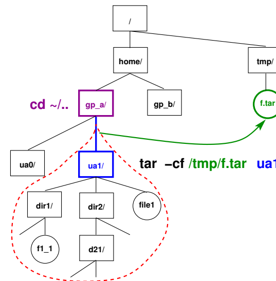
FIGURE 8 – Création (sous /tmp ) de l'archive f.tar de la branche de l'utilisateur ua1 :
