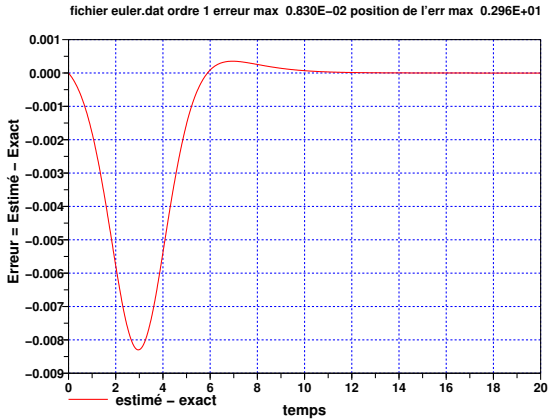
FIGURE 2 – Erreur dans l'intégration de l'équation logistique avec la méthode d'Euler pour h = 0,02 . L'allure régulière montre que l' erreur de troncature domine. Erreur de troncature locale liée à la courbure de la solution
